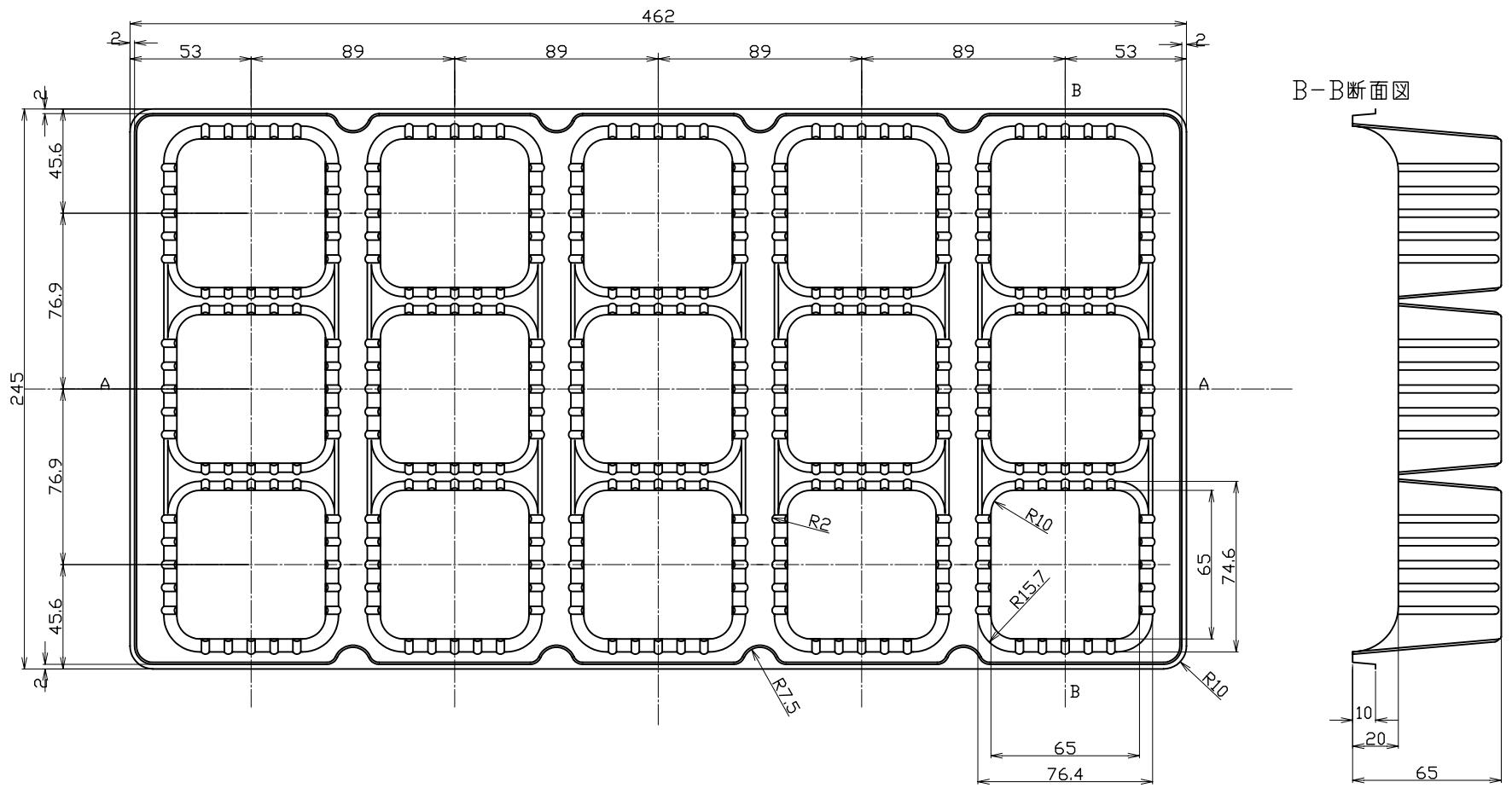
A-A断面図
