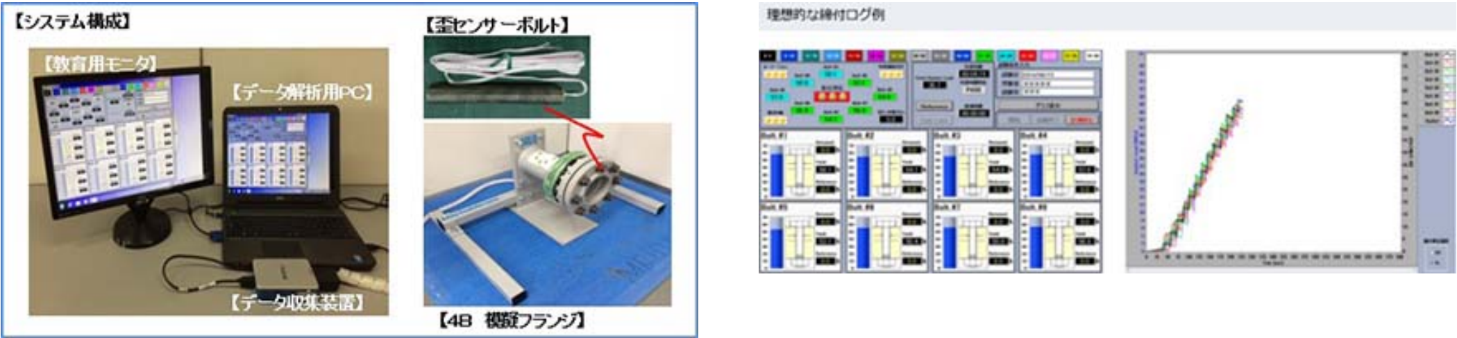
画像1 フランジボルトニングシミュレーター（D-BOLVIS: Daicel Bolting Visualization）
