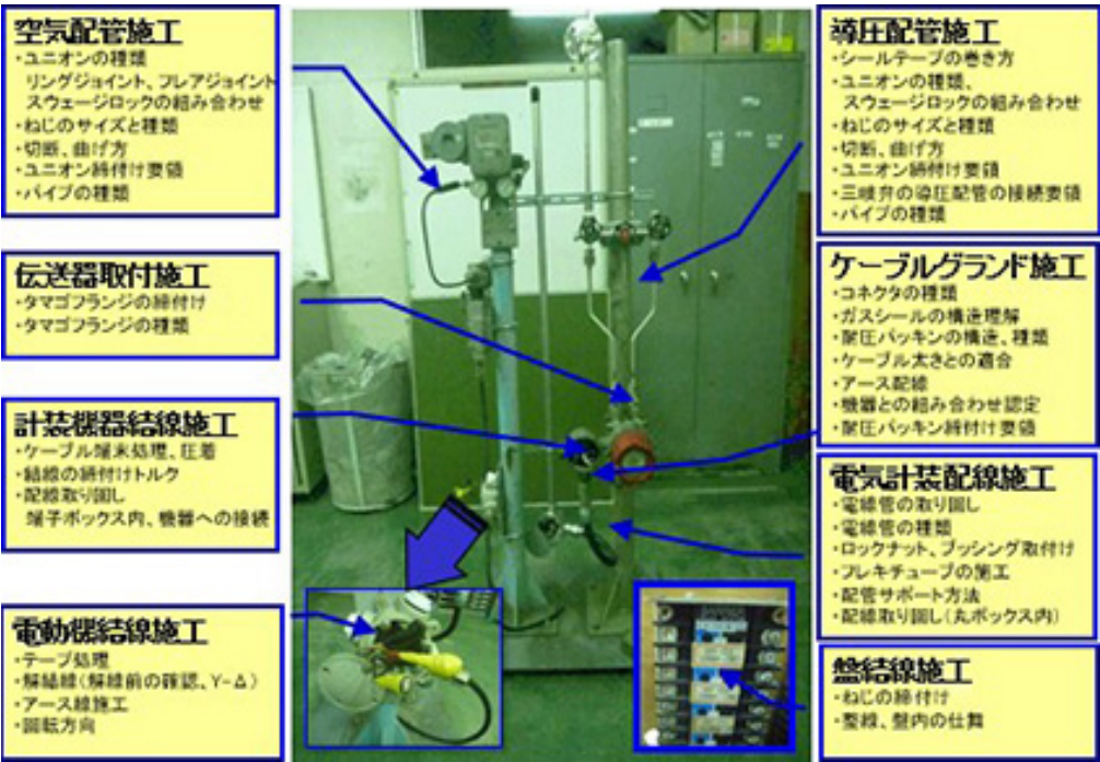
画像3 施工／製作実習用のトレーニング装置
